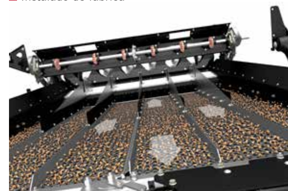
Trabajo en laderas con sistema de limpieza X Flow
